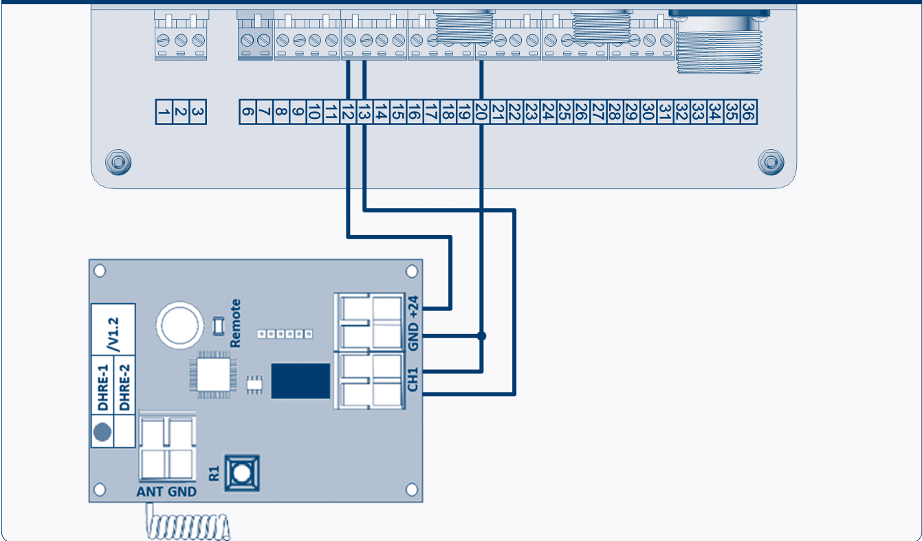
Рис. 17. Подключение внешнего радиоприемника DHRE-1
