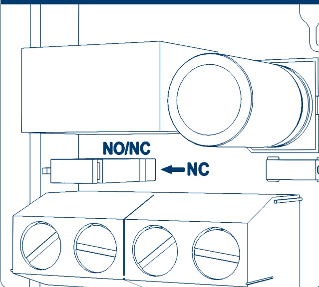
Рис. 7. Фотоэлементы. Положение переключки — NC
