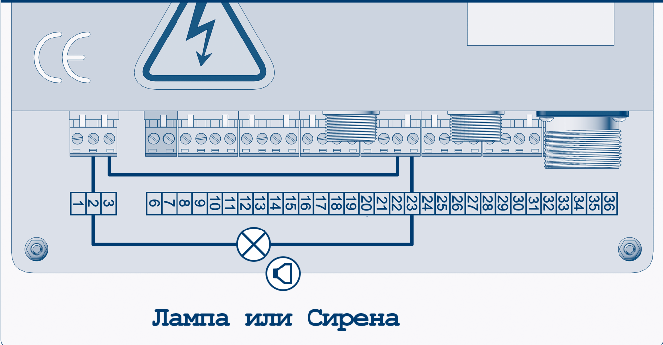
Рис. 13. Подключение сигнальной лампы или сирены 220В
