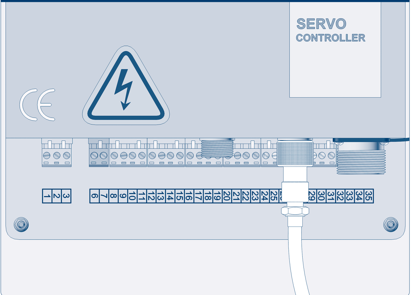
Рис. 10. Подключение внутреннего энкодера
