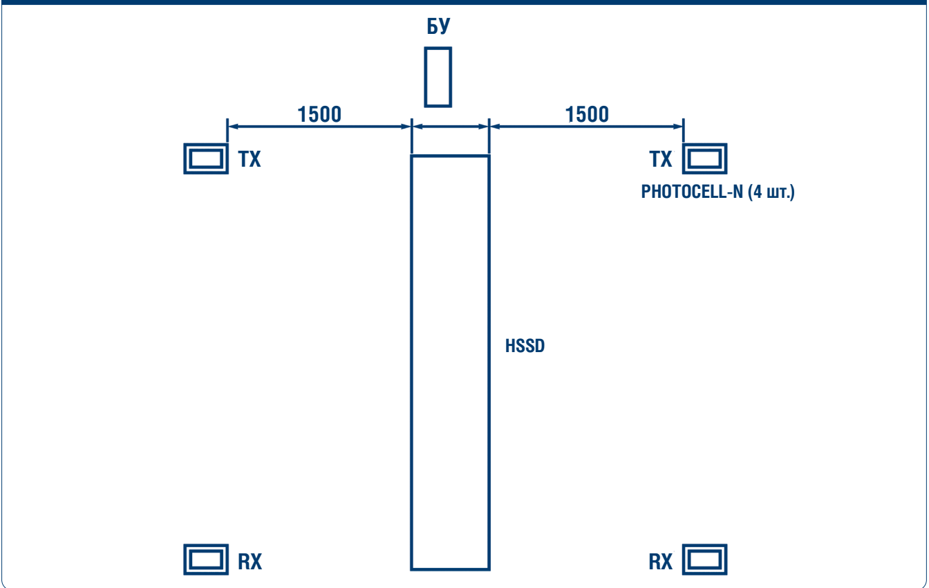
Рис. 6. Схема расположения стоек
