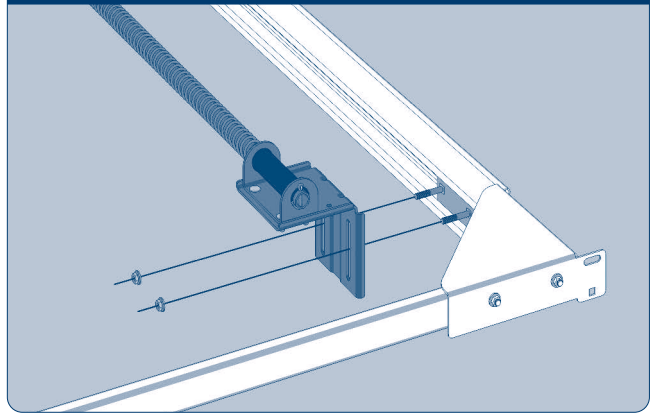
Рис. 7.7.1. Вид А
