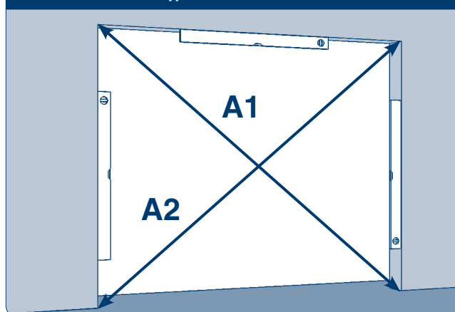
Рис. 7.1.2. Разность диагоналей
