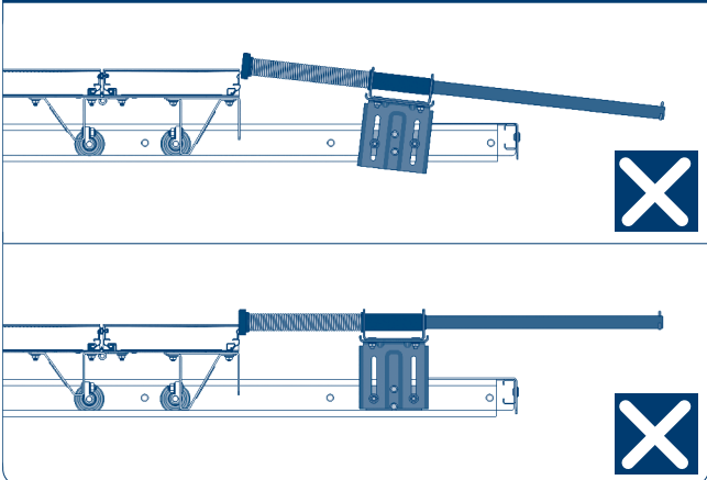
Рис. 7.7.2. Вид А (неправильно)
