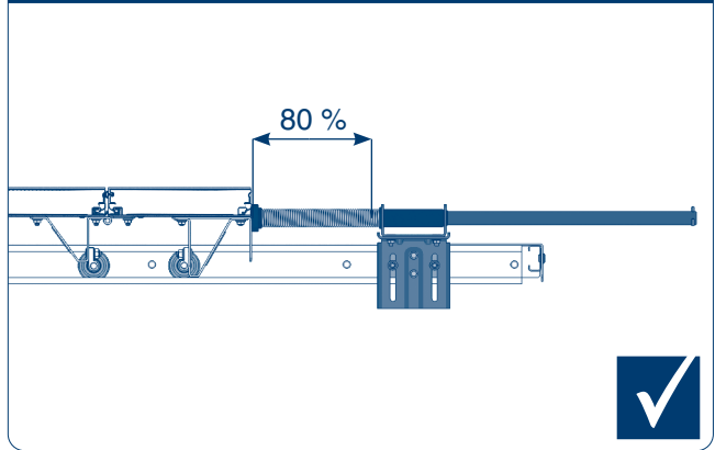
Рис. 7.7.2. Вид А (правильно)
