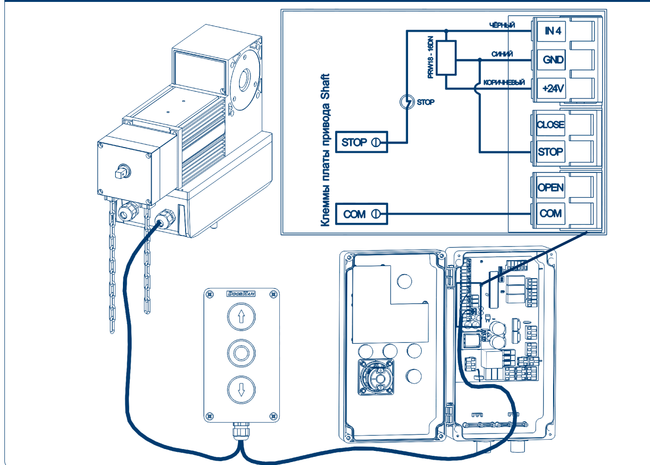
Рис. 5.1.3. Схема подключения индуктивного датчика для блоков DCUT-2
