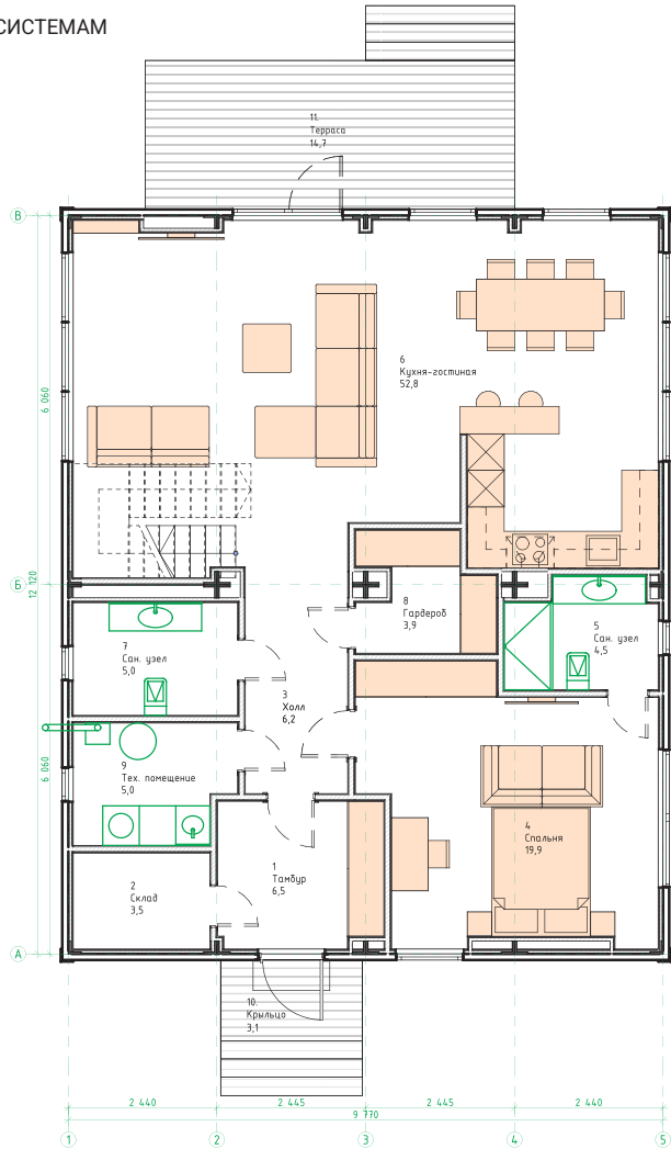
План 1-го этажа
