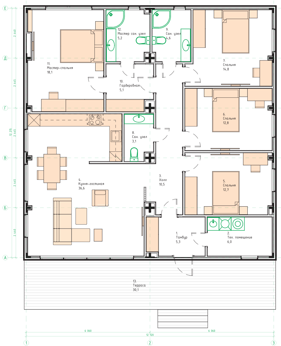
План 1-го этажа
