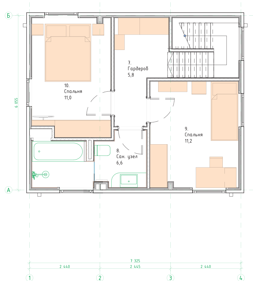
План 2-го этажа
