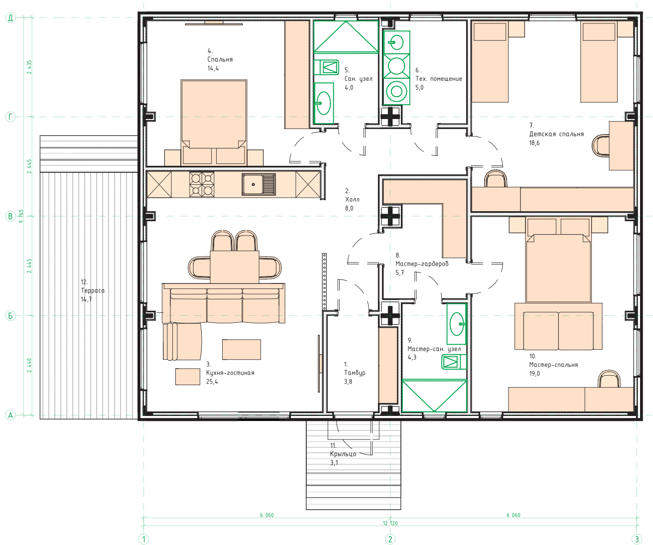
План 1-го этажа
