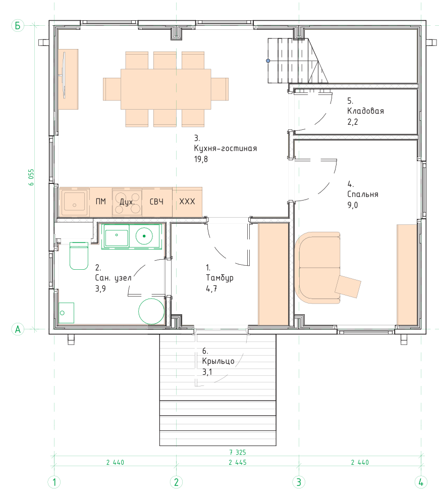
План 1-го этажа
