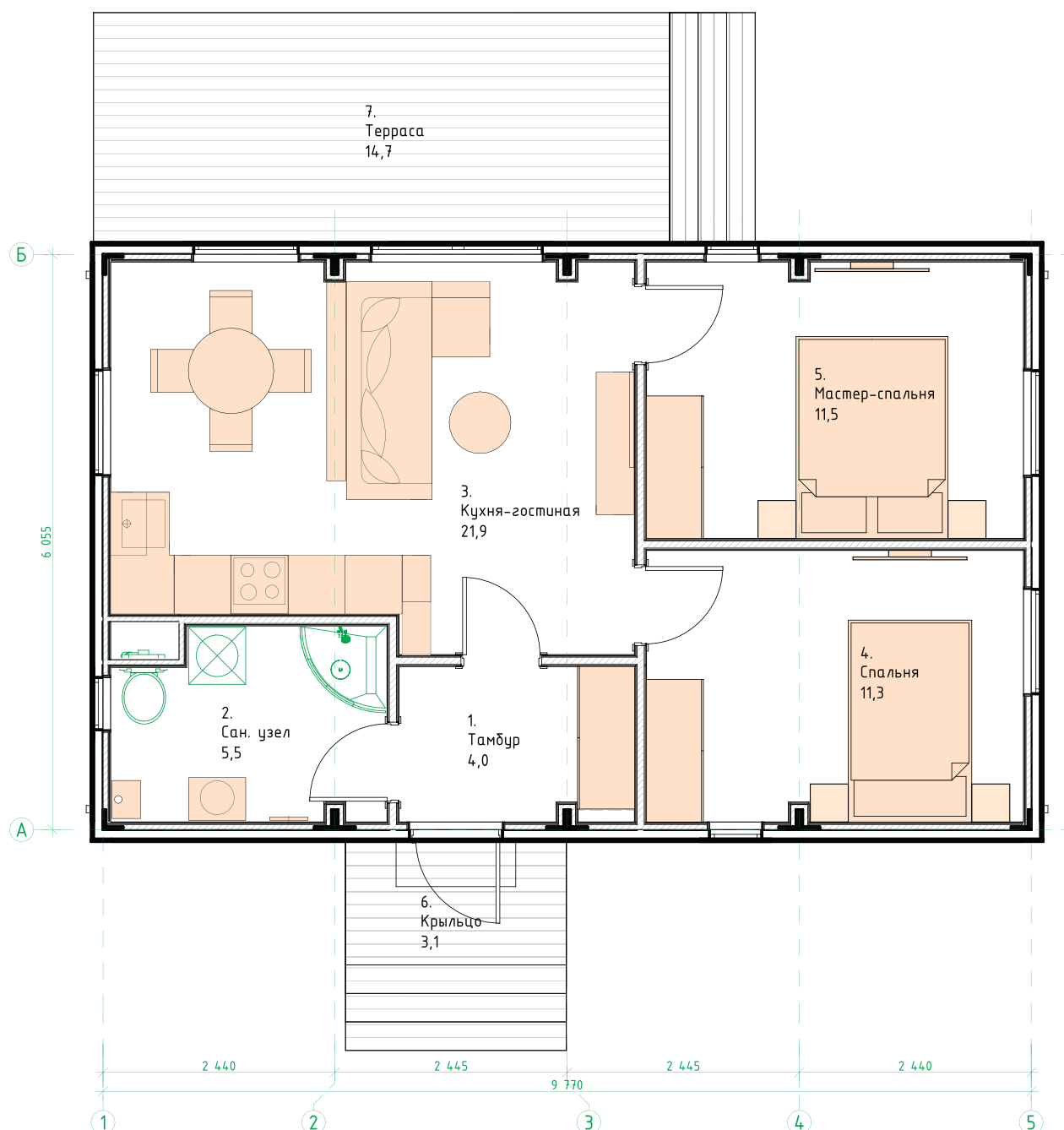
План 1-го этажа
