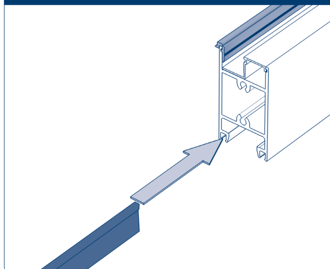
Рис. 6.2.7. Установка щетки
