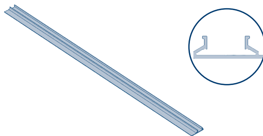
Рис. 2.6. Профиль порога «антипаника» 58 × 12 мм
