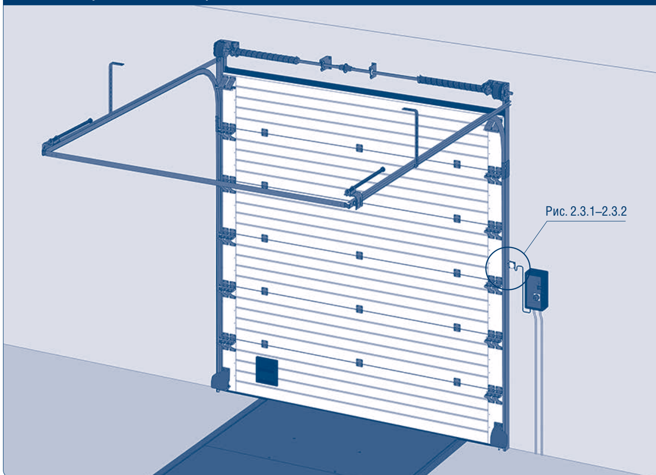
Рис. 2.3. Место установки датчика ворот E3JK-DS30M2
